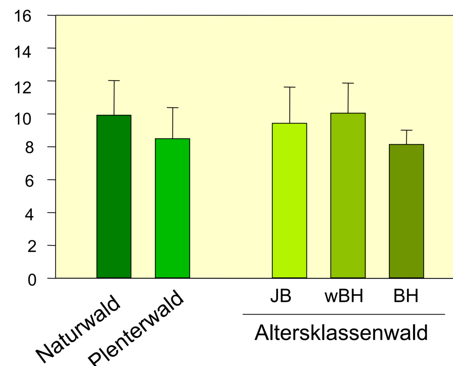
Abb.3: Gesamtvräte des org. Kohlenstoffs (OC) unter verschiedenen Landnutzungsintensitäten im Mineralboden
