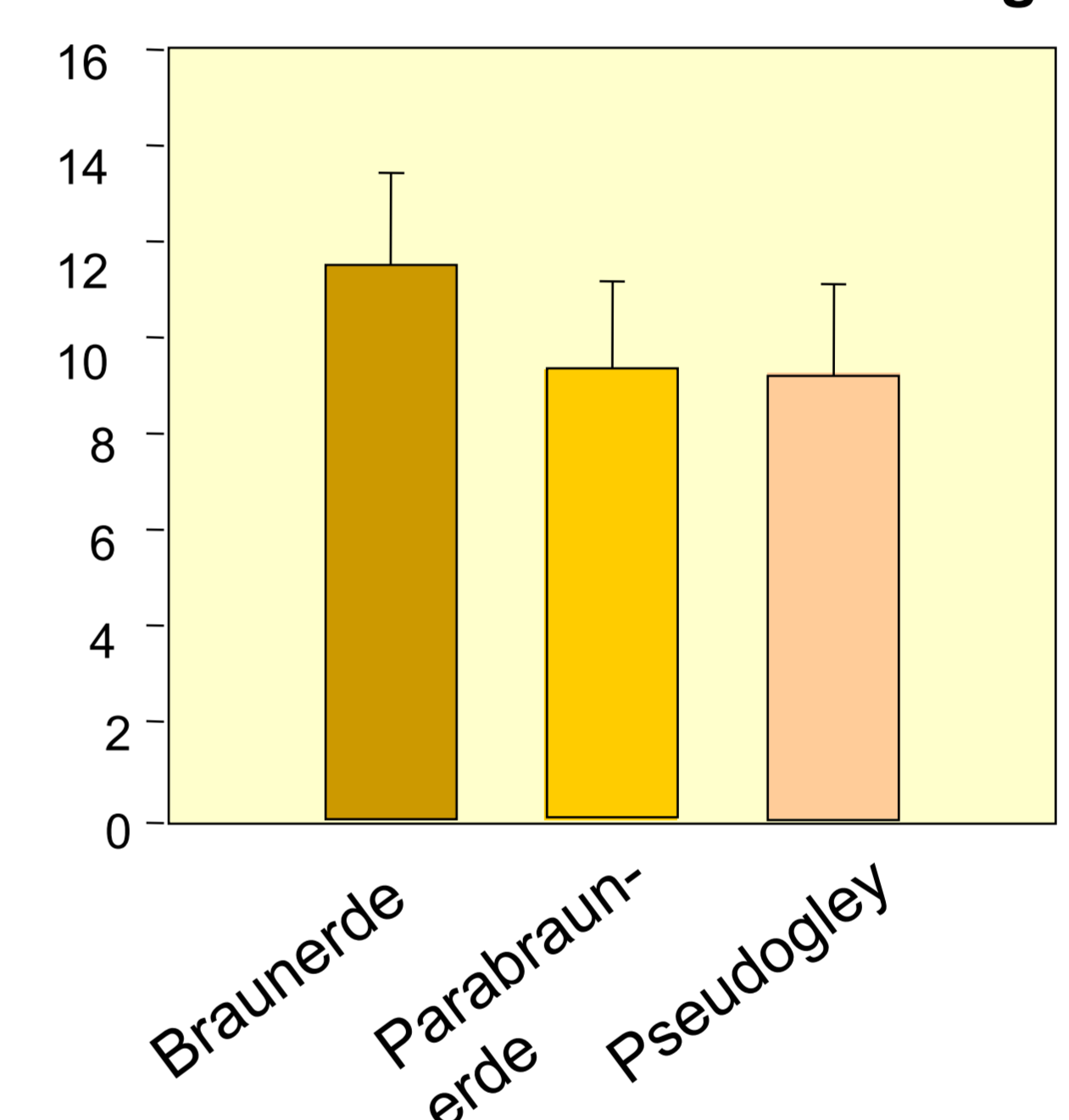
Abb.4: Gesamtvräte org. Kohlenstoffs (OC) in verschiedenen Bodentypen
