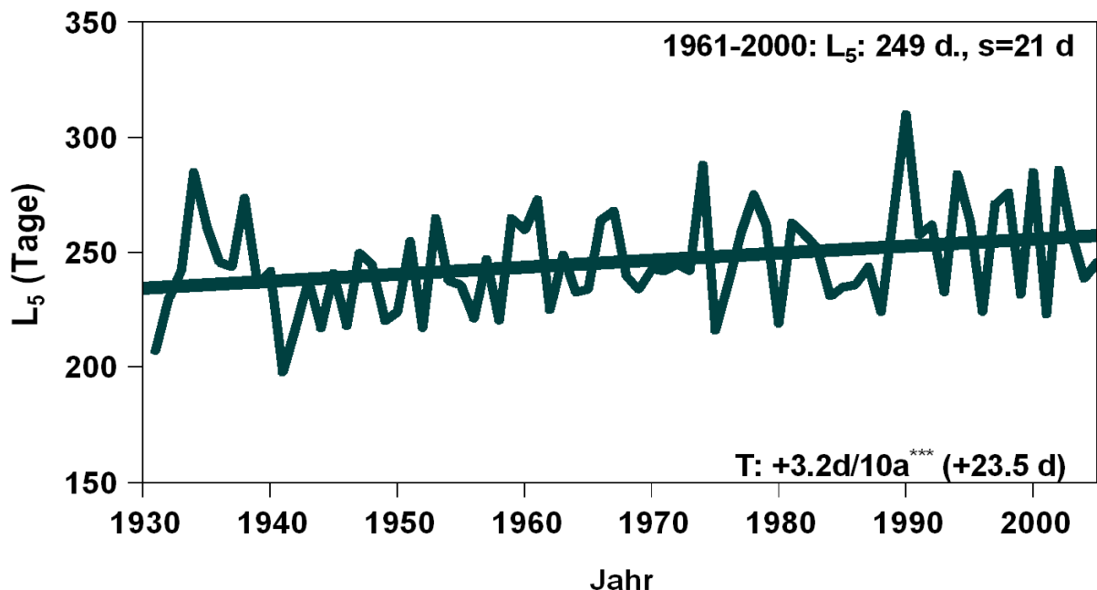
Abbildung 1: Länge der Vegetationsperiode am Standort Berlin-Dahlem (Chmielewski 2008)
