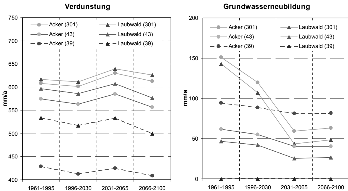
Abb. 7: Entwicklung von aktueller Evapotranspiration und Grundwasserneubildung nach WEREX IV A2 NOR (1961-2100 Chemnitz) auf Boden 301 (nFKWe 154-207 mm), Boden 43 (nFKWe 120 mm) und Boden 39 (nFKWe 50 mm)
