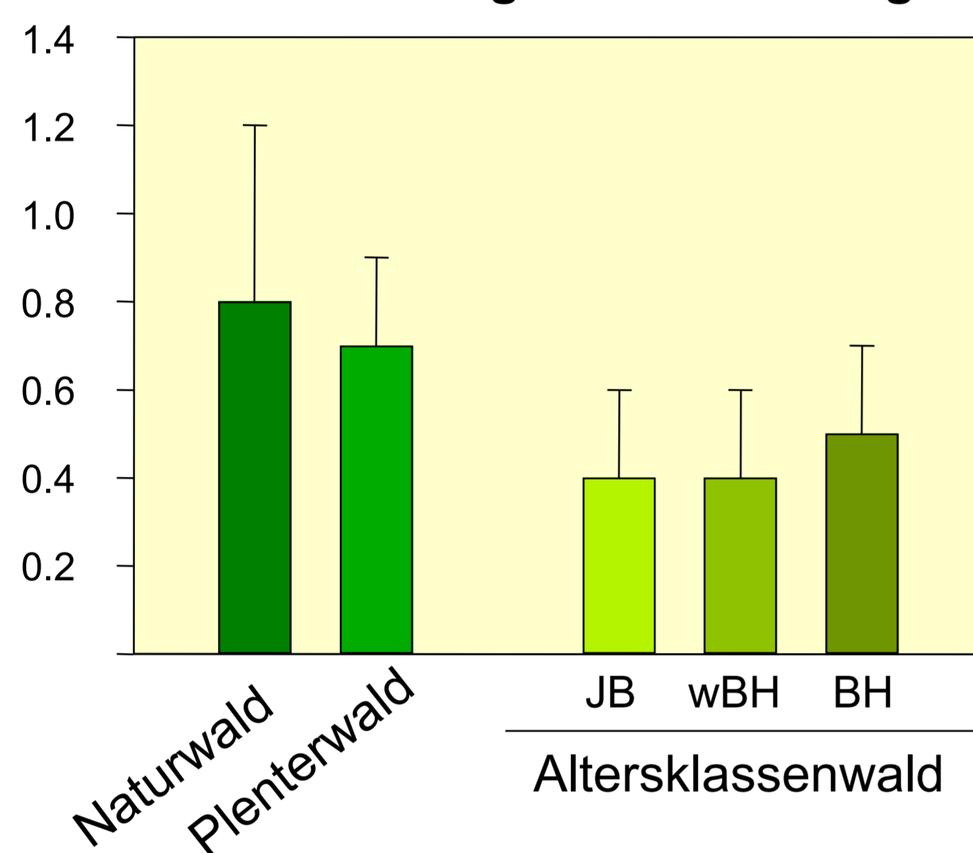
Abb.2: Gesamtvräte org. Kohlenstoffs (OC) unter verschiedenen Landnutzungsintensitäten in der organischen Auflage
