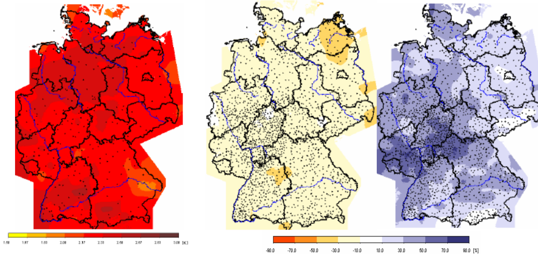
Jahresmitteltemperatur (+2,3°C) & Niederschlagsentwicklung (Sommer, -22,0%, Winter + 30,3%) im Jahr 2071-2100 nach IPCC-SRES A1B (Basis 1961-1990; Spekat, et al. 2007)
