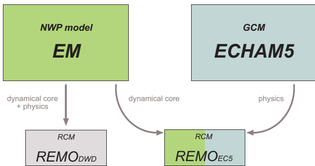
Abb. 2: Das regionale Klimamodell REMO_{EC5} (nach: URL http://www.mpimet.mpg.de/wissenschaft/ueberblick/atmosphaere-im-erdsystem/regionale-klimamodellierung/the-remo-model/the-regional-model-remo.html )
