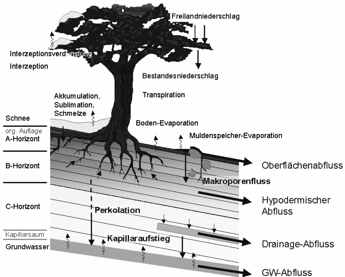
Abb. 1: Wasserflüsse und Teilglieder des Wasserhaushaltes in ArcEGMO
