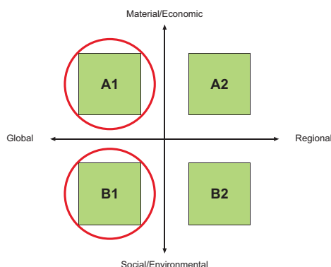
Abb. 3: SRES-Szenarien (IPCC 2001, 2007)
